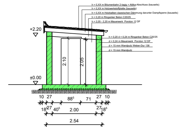
Kleintierhaus - Schnitt AA
