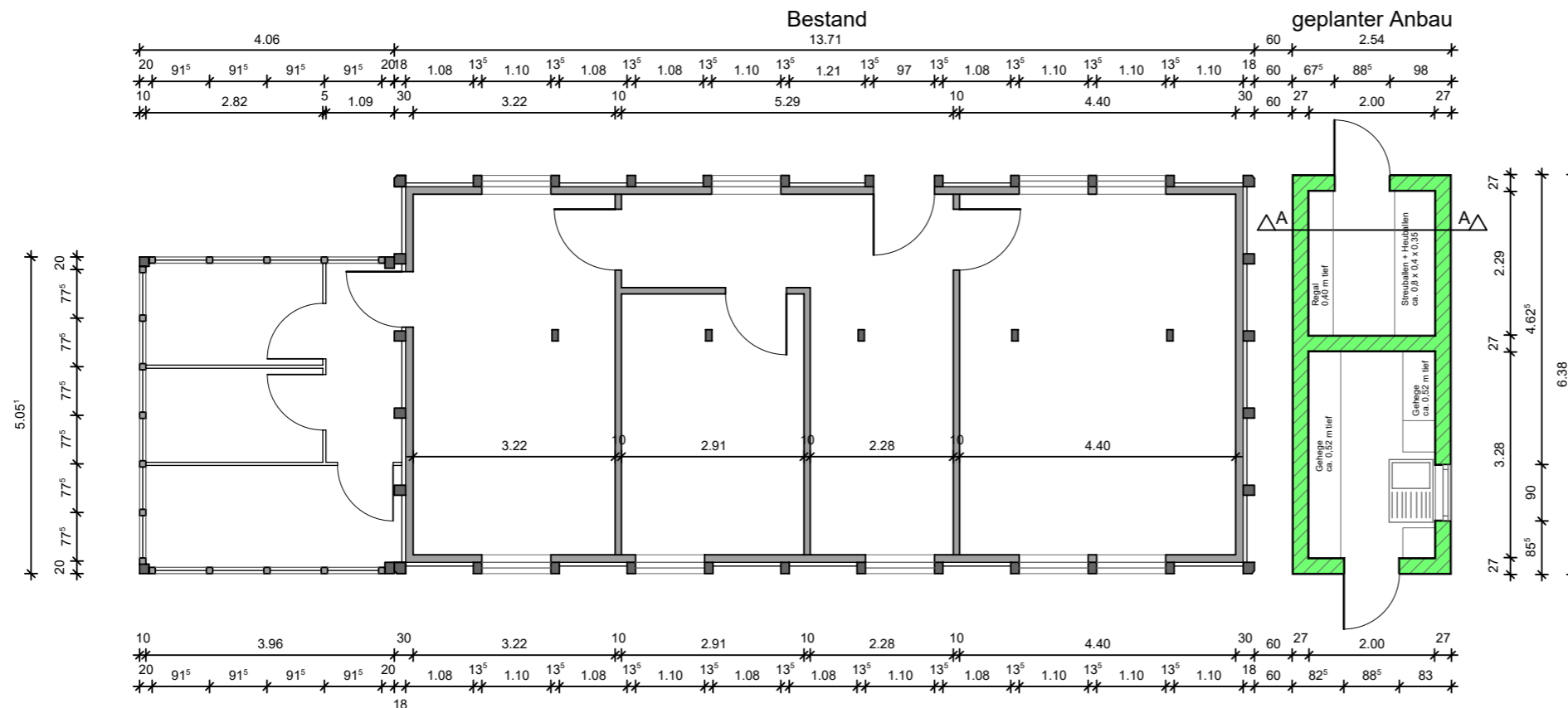
Kleintierhaus - Grundriss
